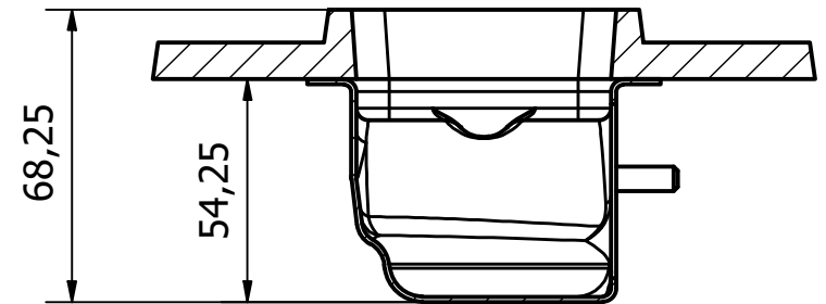
A-A ( 1/2 )
